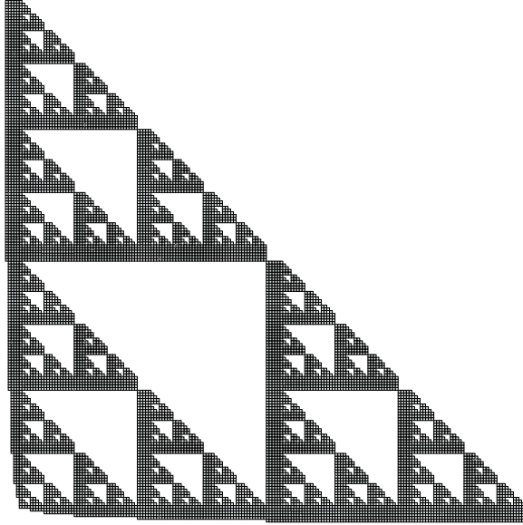
Fig. 2. Fibered Sierpinski Triangle T
